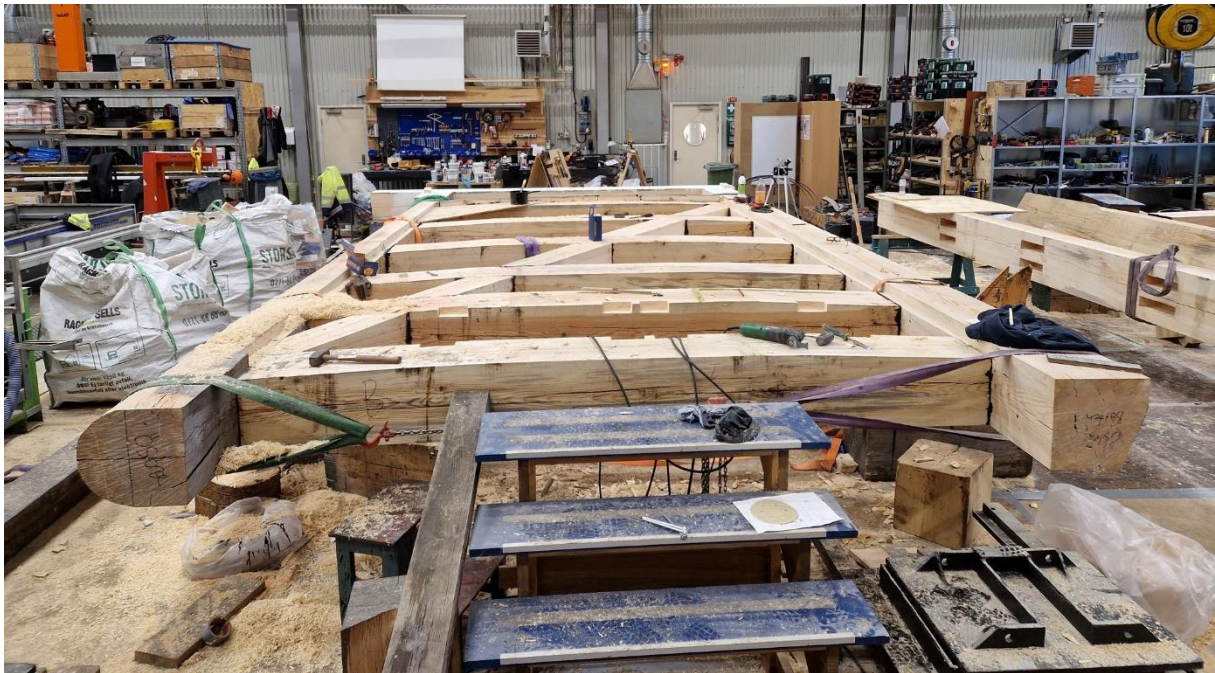
Sörkvarns slussport, februari 2025, verkstaden i Hallstahammar. Foto: Hans-Lennart Ohlsson
